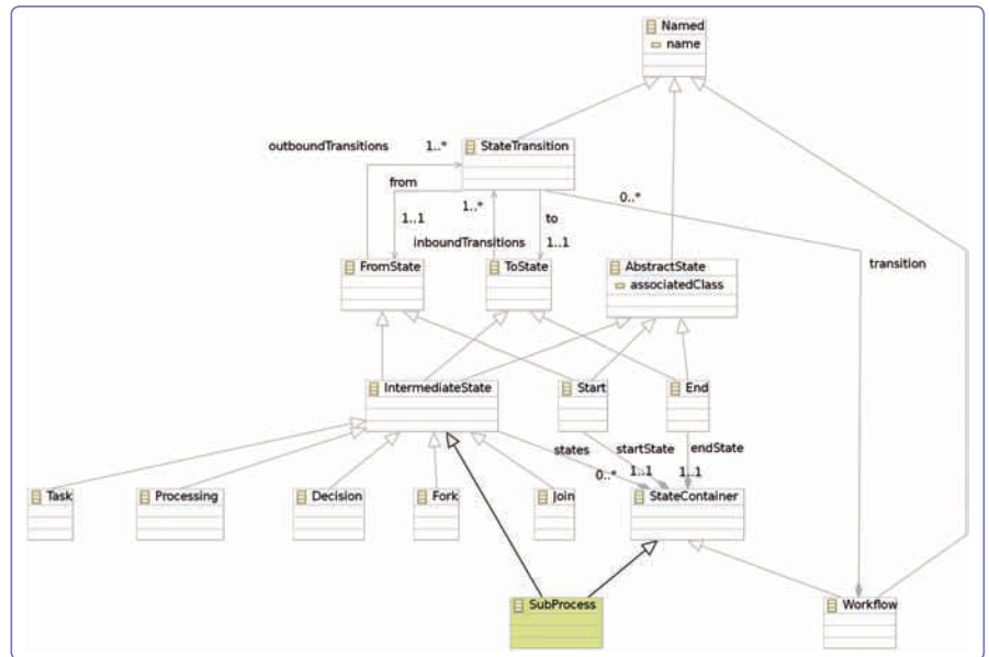
Abb. 1: Erweitertes Workflow-Metamodell
